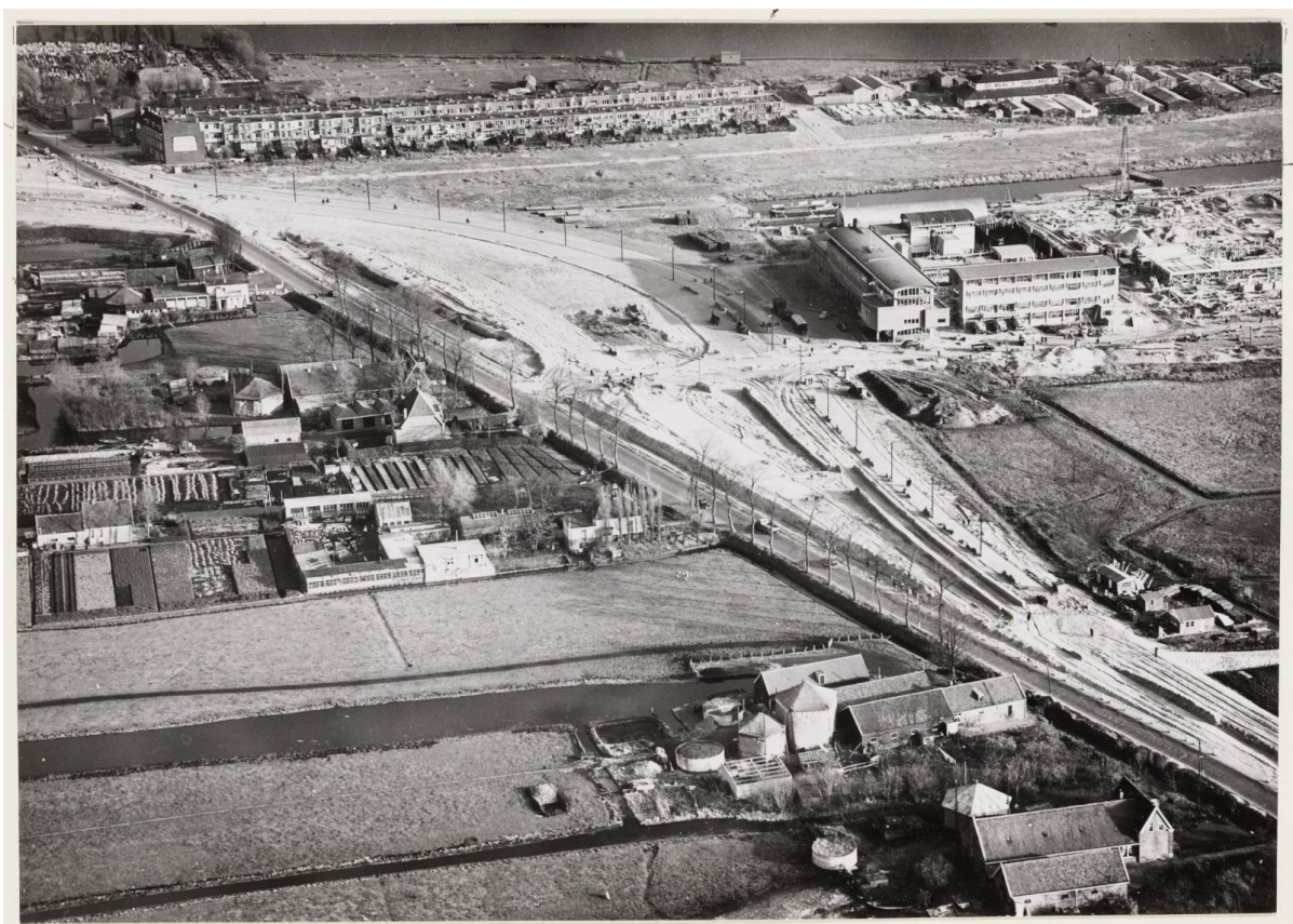
16 november 1948: Het oude tracé van de Sloterweg, langs de huizen en boerderijen op de voorgrond, is nog zichtbaar. De verbreding, met de ruime boog richting het Aalsmeerplein, langs het toen nog nieuwe Nationaal Luchtvaartlaboratorium, is nog in aanleg. Foto: Beeldbank Stadsarchief Amsterdam.
